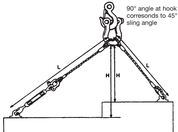
45^\circ SLING ANGLE
